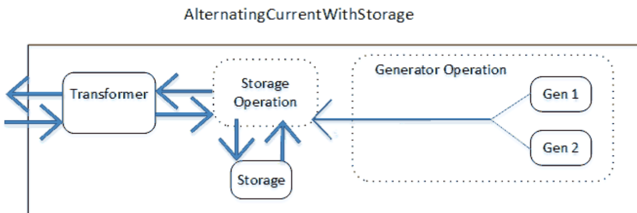
Figure 1.208: LoadCenterBussType
